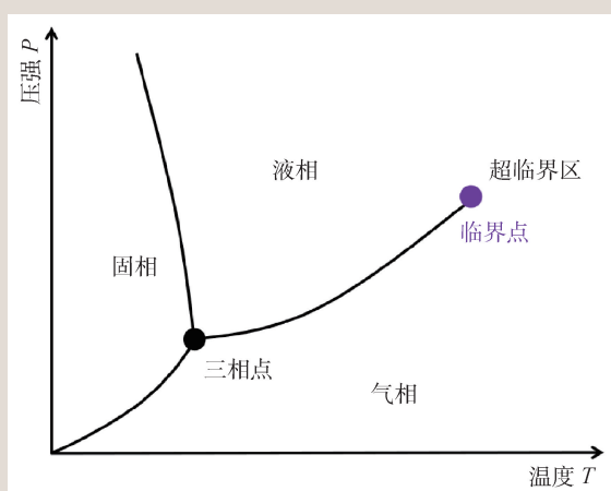
图1 水的相图
