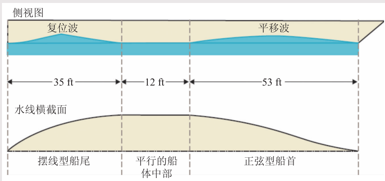
图2 波形线理论规定了3个主要船体几何参数：船首采用正弦波形式，船尾采用摆线波形式，船体中间部分采用平直并与中心线平行的方式。船首和船尾的长度与相应的正弦波和摆线波波长一致，船体中间长度根据船体总长的需要调整
